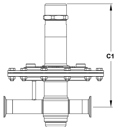
Optional top cap
