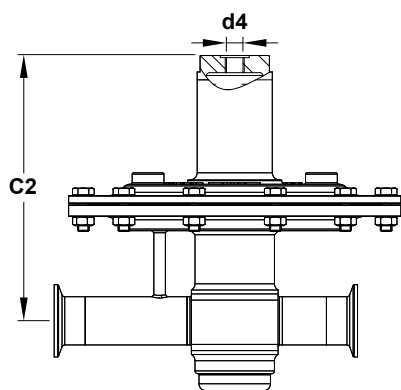
Optional dome-loading
